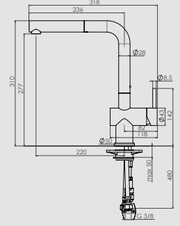
Tek-kumanda kollu çıkartılabilir başlıklı armatür LIVE
